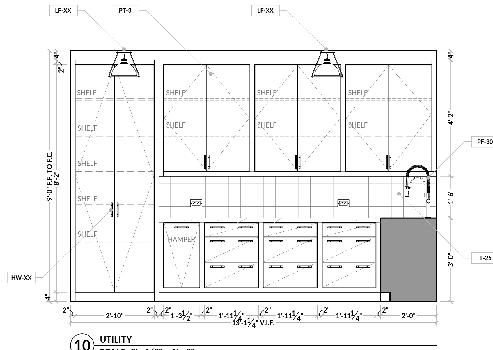
10 UTILITY SCALE: 0' - 1/2" = 1' - 0"
