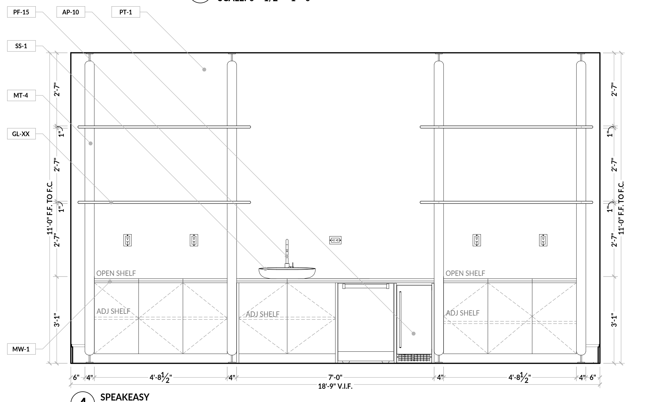
4 SPEAKEASY SCALE: 0' - 1/2" = 1' - 0"
