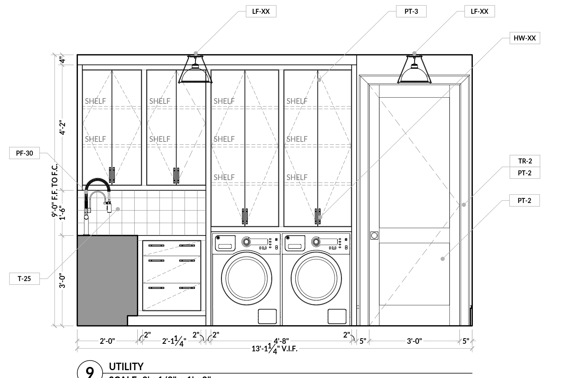
9 UTILITY SCALE: 0' - 1/2" = 1' - 0"
