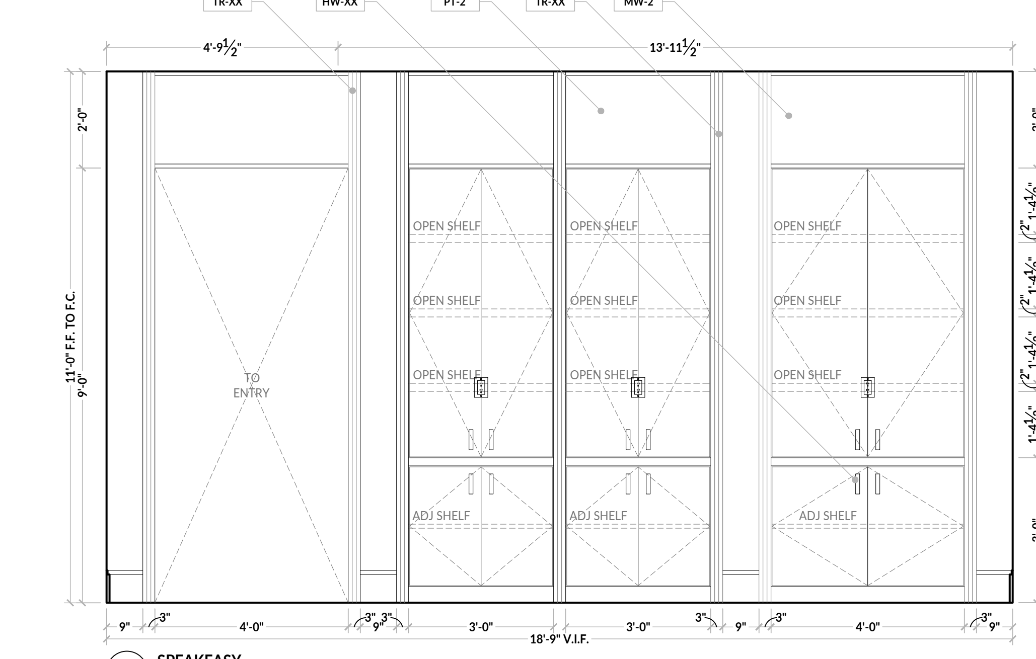
3 SPEAKEASY SCALE: 0' - 1/2" = 1' - 0"
