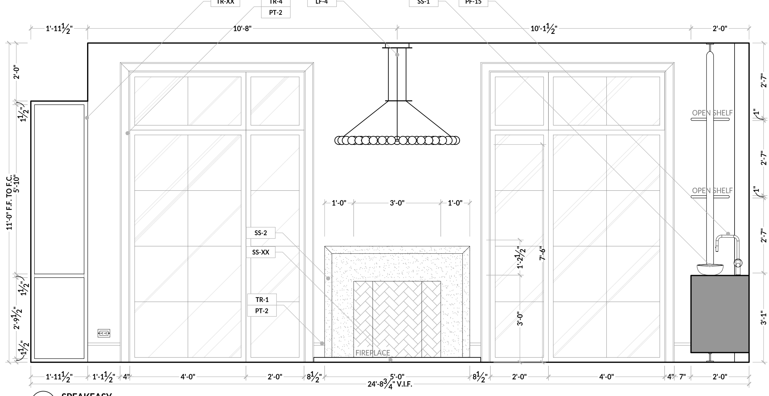
1 SPEAKEASY SCALE: 0' - 1/2" = 1' - 0"
