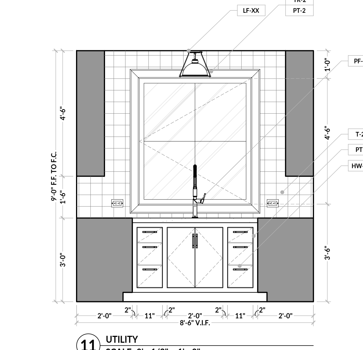
11 UTILITY SCALE: 0' - 1/2" = 1' - 0"
