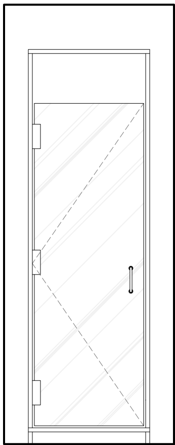
6 BATHROOM 3 SCALE: 0' - 1/2" = 1' - 0"
