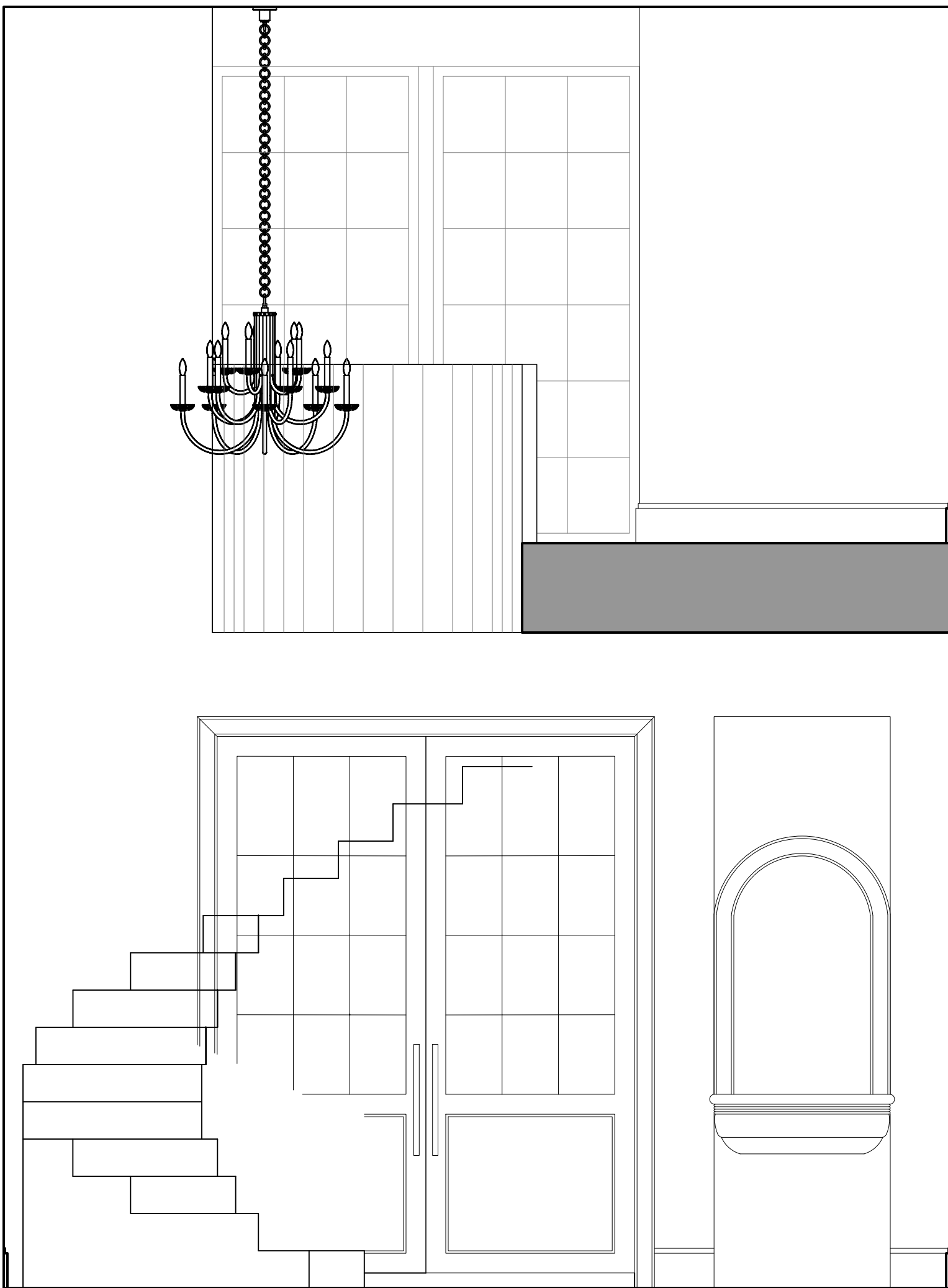
1 FOYER SCALE: 0' - 1/2" = 1' - 0"
