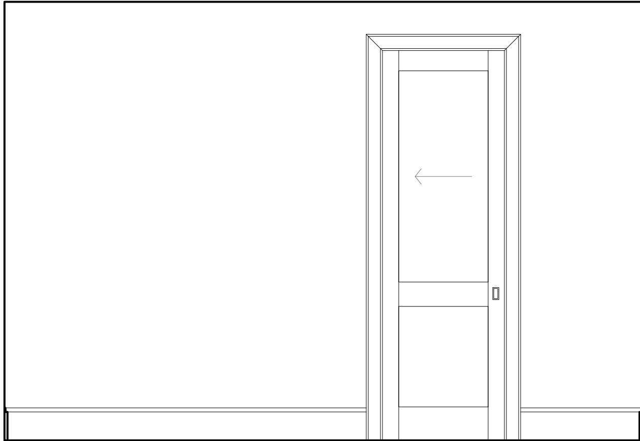
5 BEDROOM 1 SCALE: 0' - 1/2" = 1' - 0"
