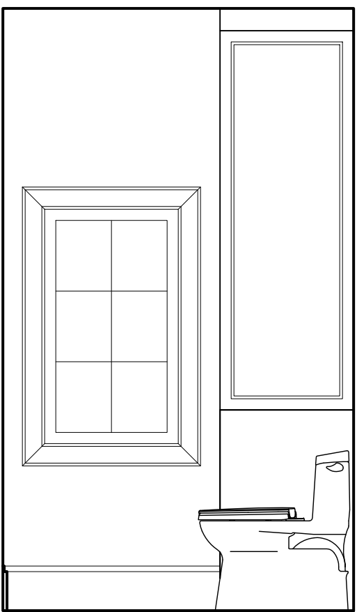
5 BATHROOM 2 SCALE: 0' - 1/2" = 1' - 0"
