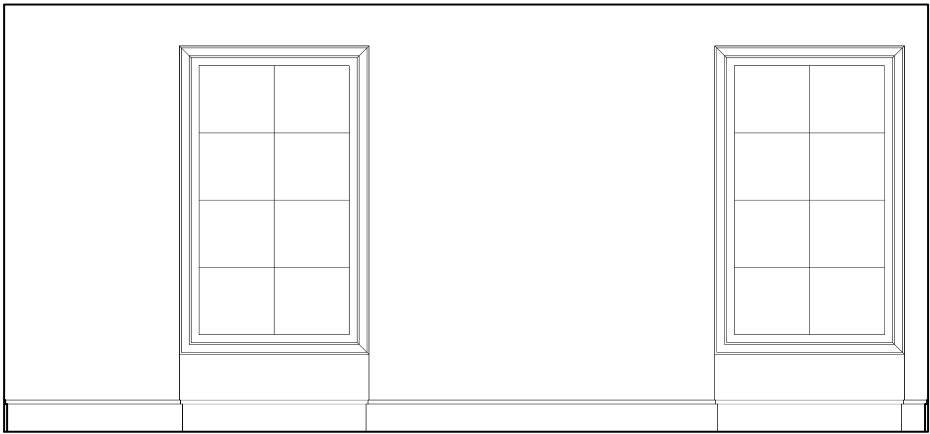
10 GYM SCALE: 0' - 1/2" = 1' - 0"
