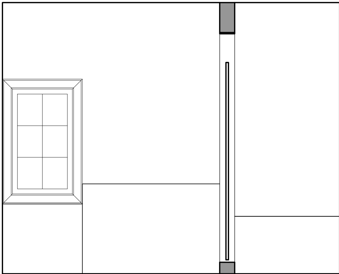
13 BATHROOM 3 SCALE: 0' - 1/2" = 1' - 0"
