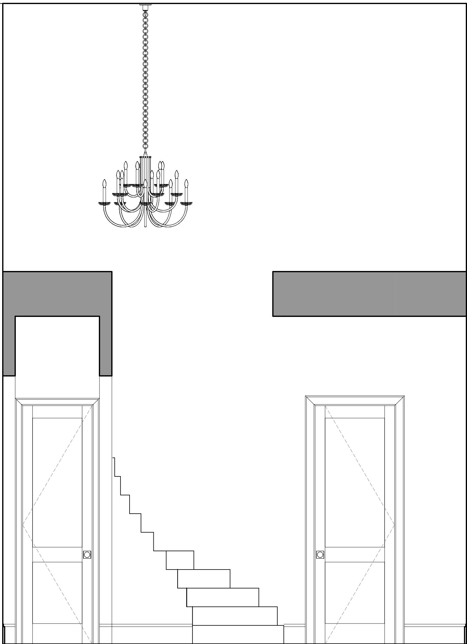
3 FOYER SCALE: 0' - 1/2" = 1' - 0"
