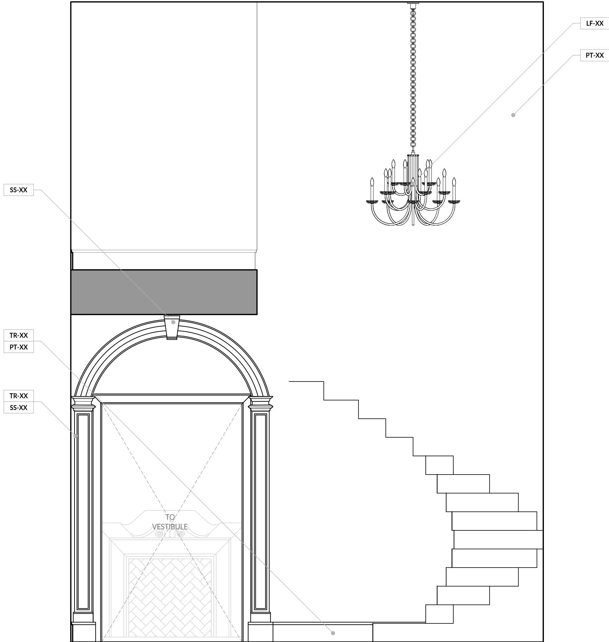
1 FOYER SCALE: 0' - 1/2" = 1' - 0"
