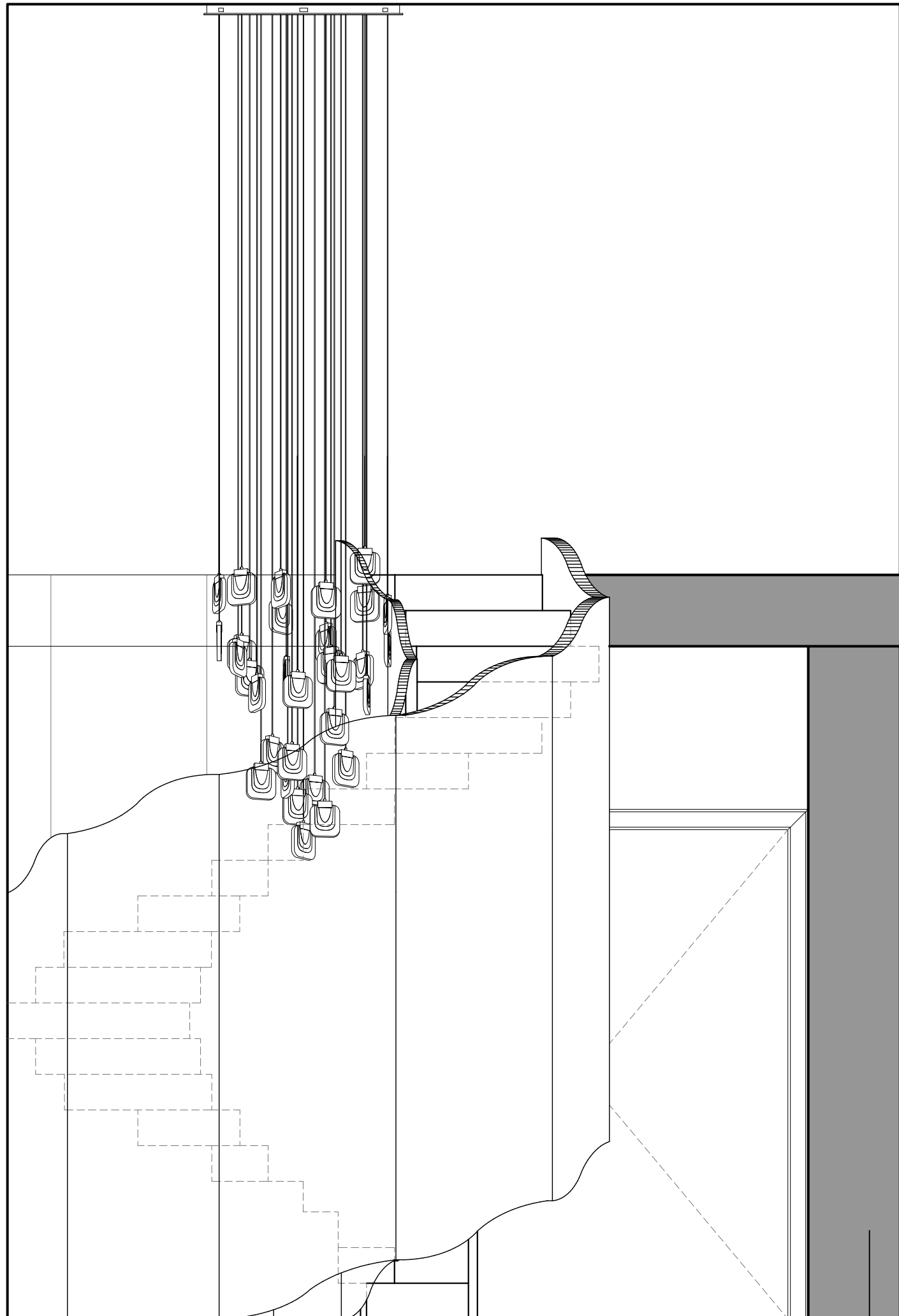
1 MUDROOM SCALE: 0' - 1/2" = 1' - 0"
